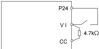
<源极逻辑>
