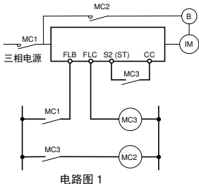
电路图 1
