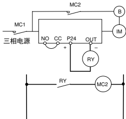
电路图 2
