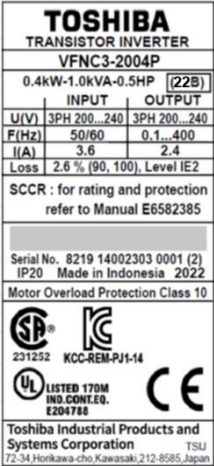
定格銘板例
