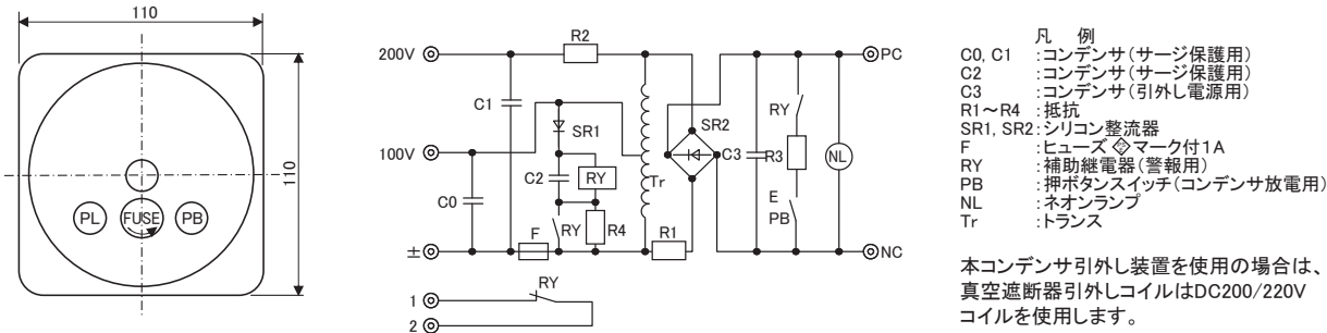
第30図 コンデンサ引外し装置CIT-10Q
