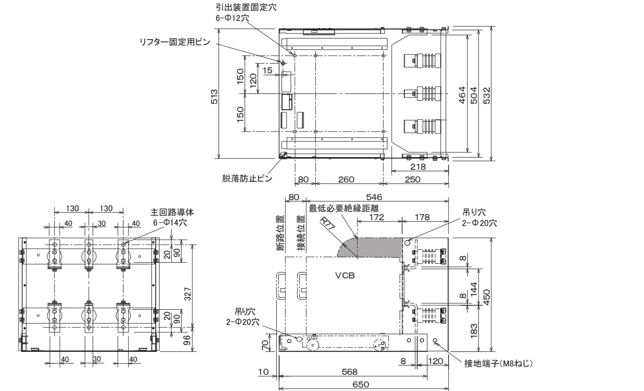
第11図 U6A-VL1形水平引出装置外形寸法図(導体方向垂直)
