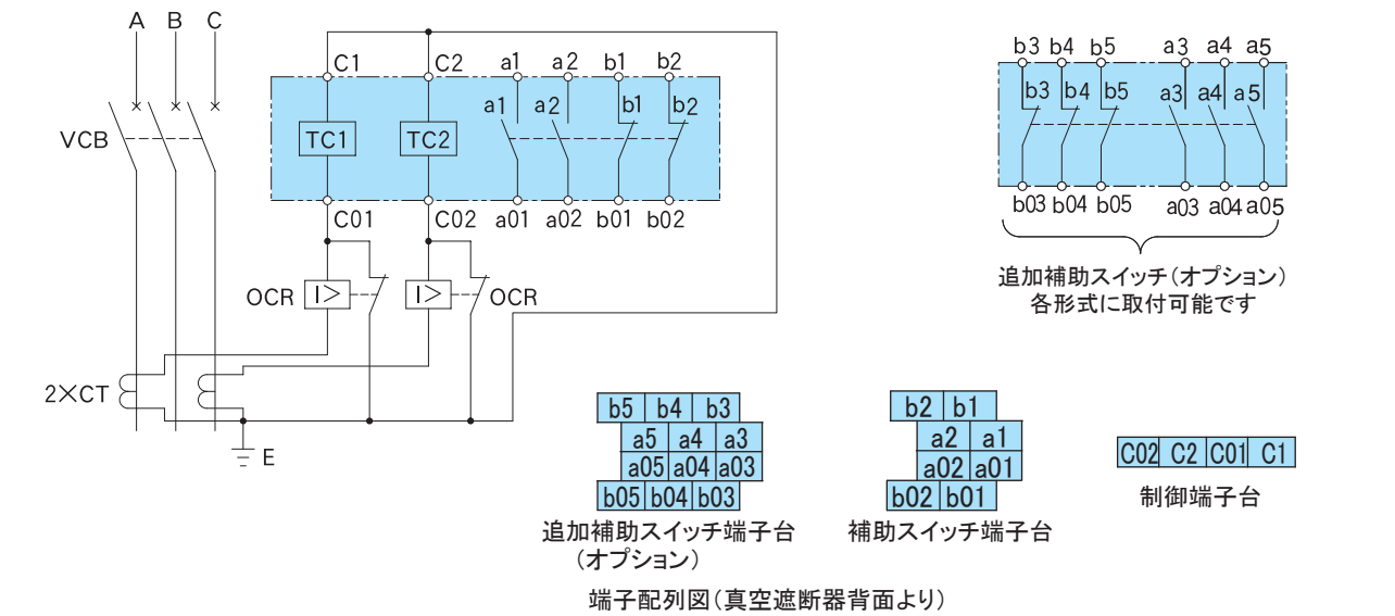
(a) CT二次電流引外し方式
