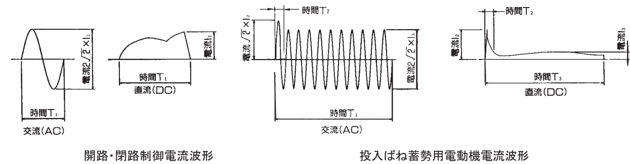
第44図 電流波形
