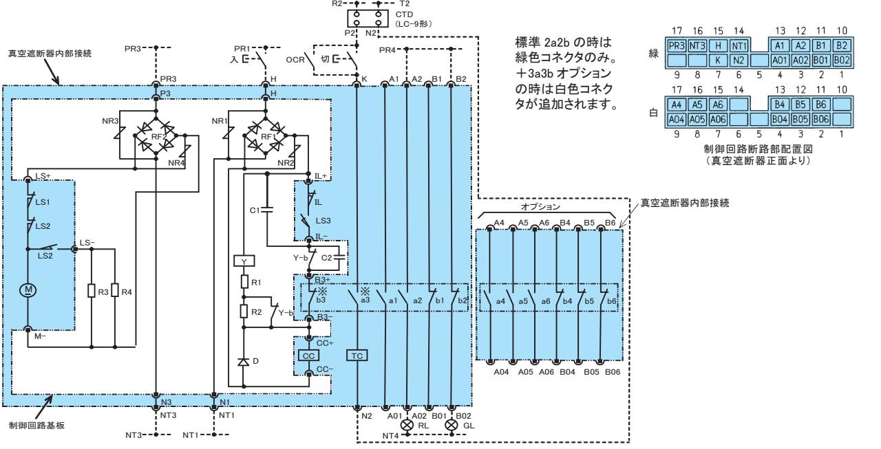
(b) コンデンサ引外し方式
