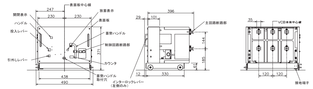
第9图 V□D(S)-MLD形水平引出形真空遮断器外形寸法图
