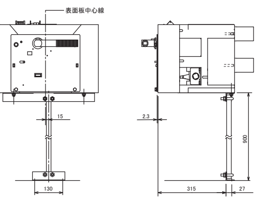
第15図 V□C(S)-L支持パイプ取付図(電動ばね操作V□D(S)-L形も同じ)
