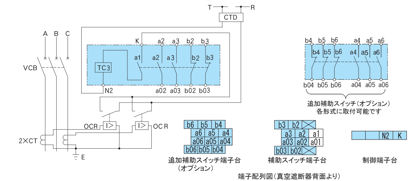
(c) コンデンサ引外し方式
