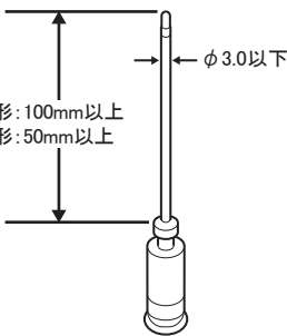
第28図 推奨油差し
