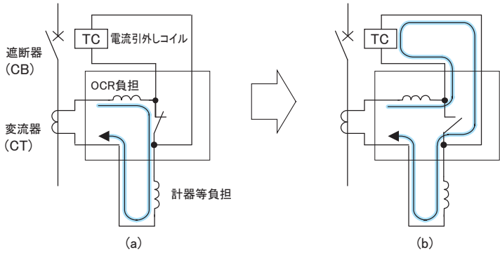
第1図 CT二次電流による遮断器動作説明
