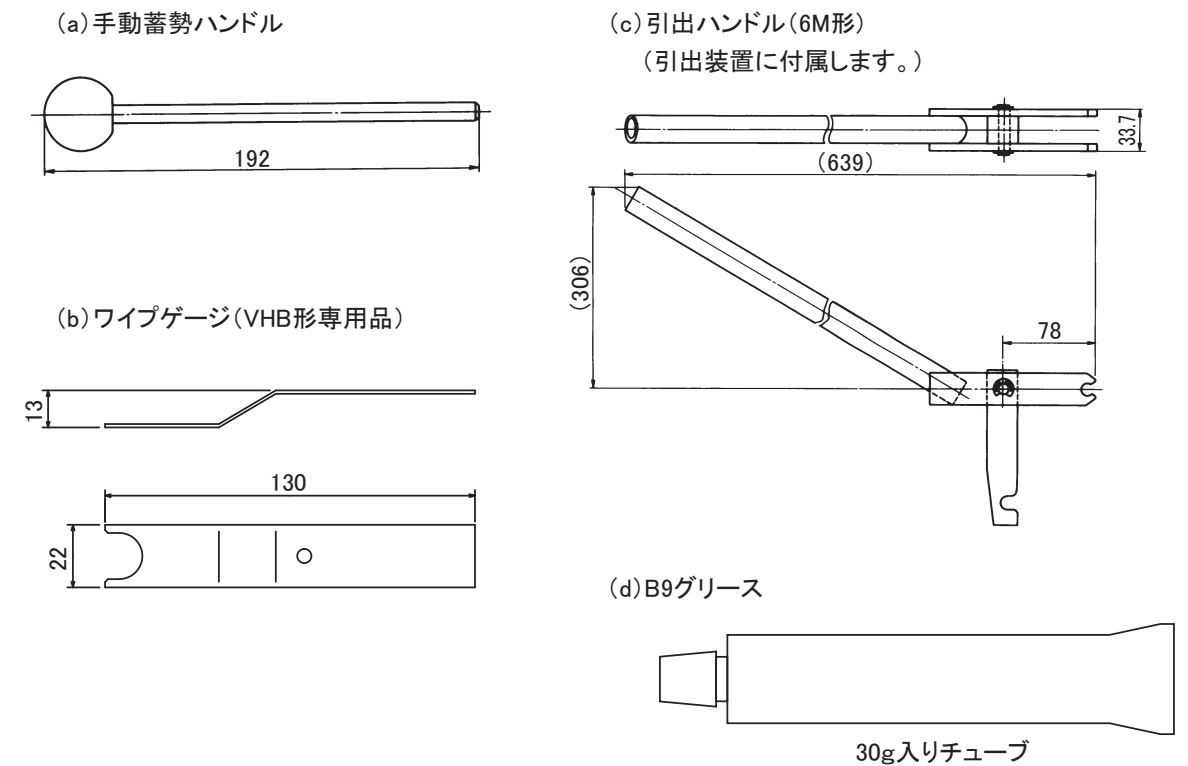
第 26 図 標準付属品
