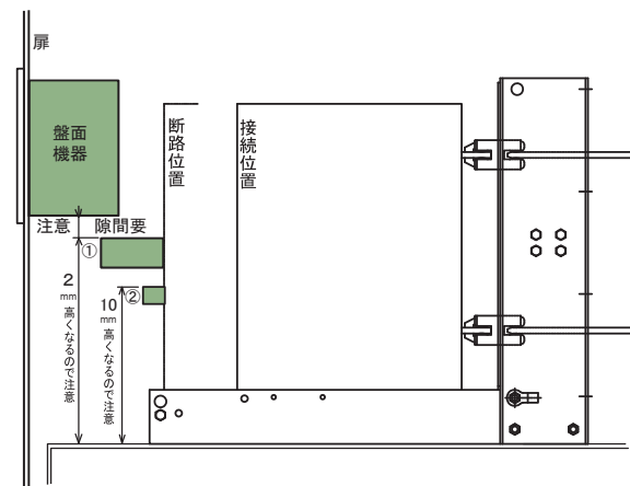
第 47 図 VHB-6J13S(VHB-6H8S,VHB-6J20S)突出部と盤面機器
