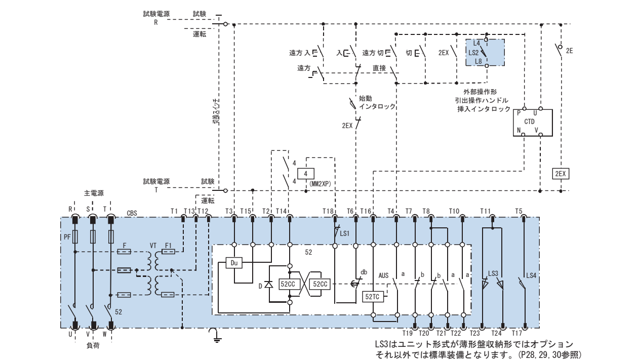
第37図 UVA形瞬時励磁式(ラッチ式)真空コンビネーションユニット展開接続図
