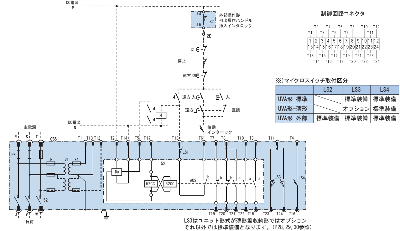
第36図 UVA形常時励磁式真空コンビネーションユニット展開接続図
