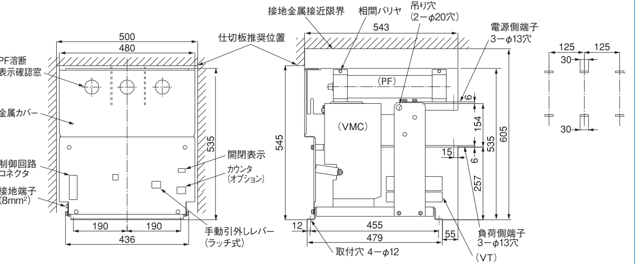
第39図 UVA形ヒューズ付真空コンタクタ外形寸法図
