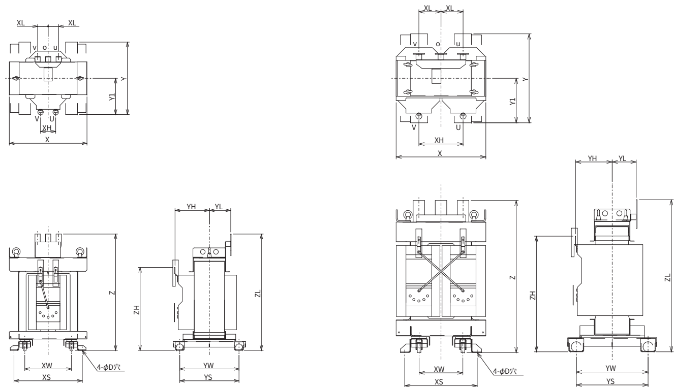
図3 10~75kVA
