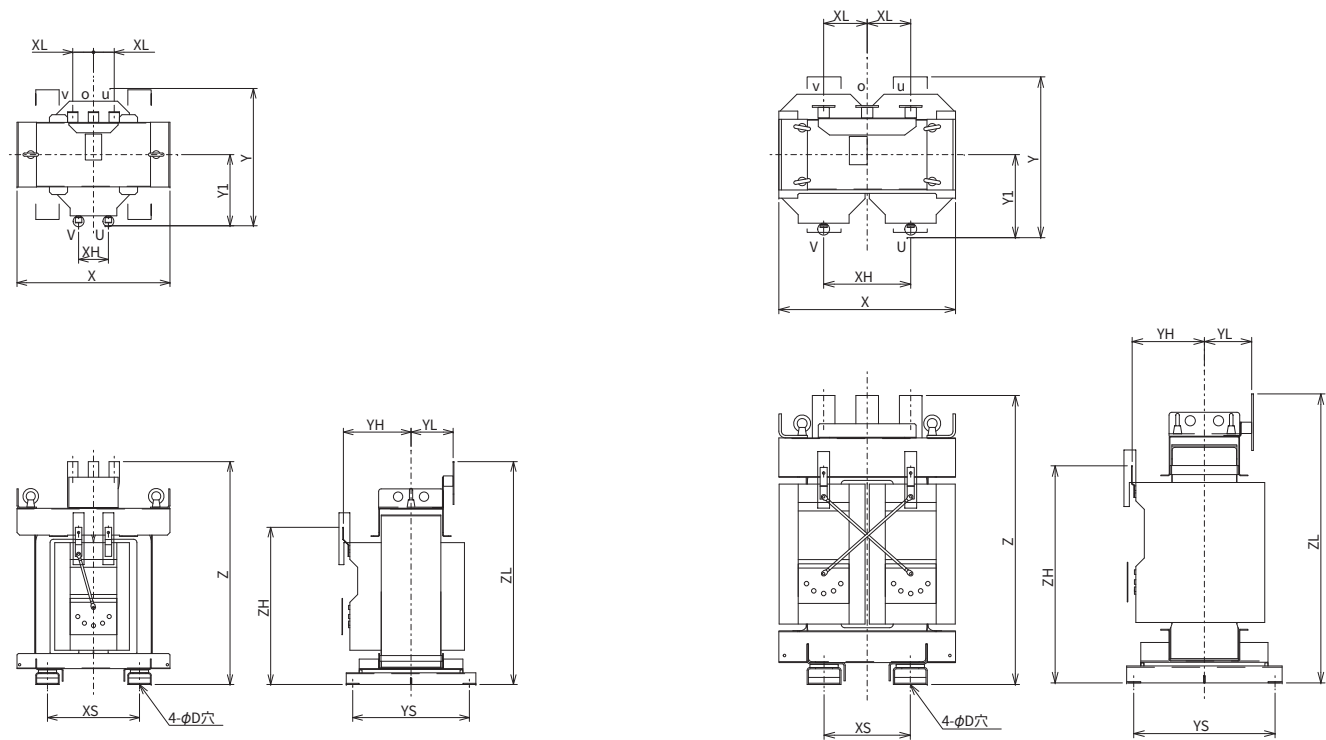
図1 10~75kVA
