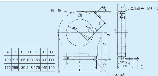
図1 AZ-ECA形
