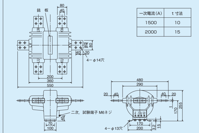
図4 ATZ-E6A形 (1500, 2000A)
