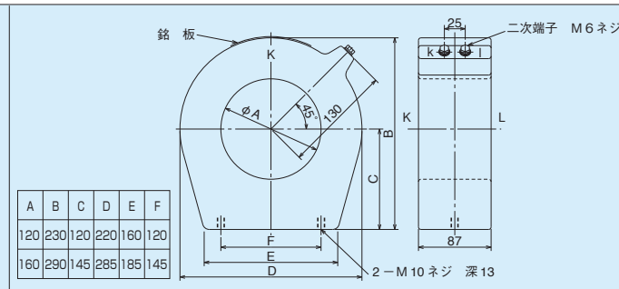
図2 AZ-ECB形
