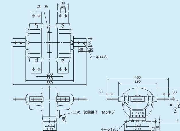
図3 ATZ-E6A形 (800A以下)
