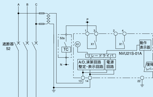
第8-4-3図 NVU21S形 外部接続図
