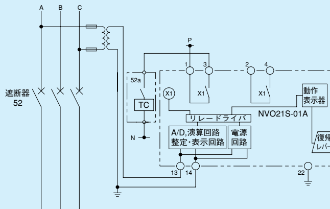
第8-3-3図 NVO21S形 外部接続図
