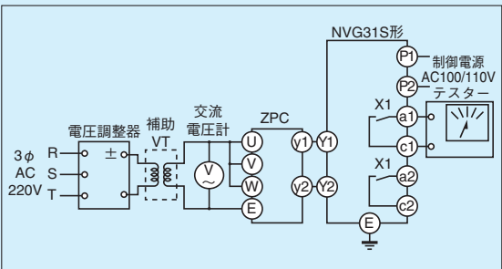
第12-8-1図 動作値試験回路
