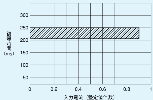
第7-8-3図 復帰時間特性
