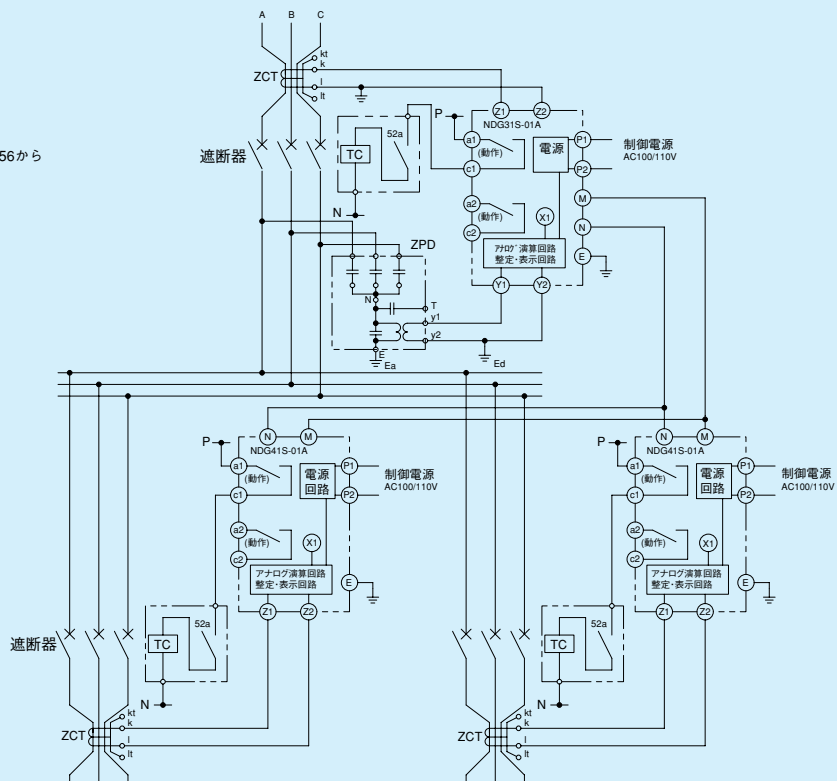
第8-8-3図 NDG31S-01A形、NDG41S-01A形 外部接続図
