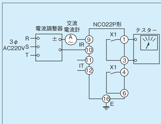
第12-2-3図 動作値試験回路
