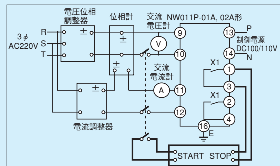
第11-10-2図 時間特性試験回路
