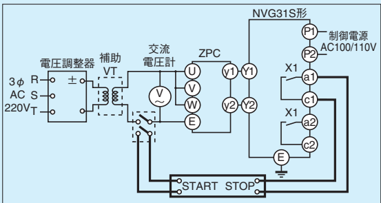
第12-8-2図 時間特性試験回路
