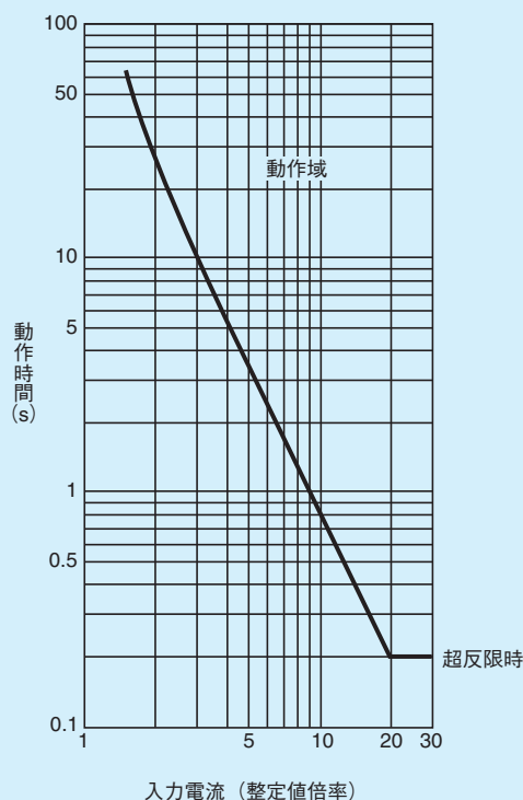
第8-2-1図 動作時間特性(限時要素)
