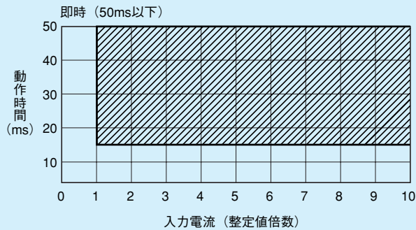
第7-6-1図 動作時間特性
