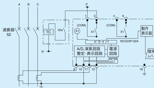
第8-1-4図 NC022P形 外部接続図
