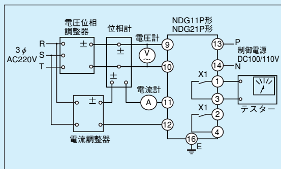
第11-8-1図 動作値試験回路
