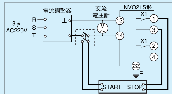
第12-4-2図 時間特性試験回路
