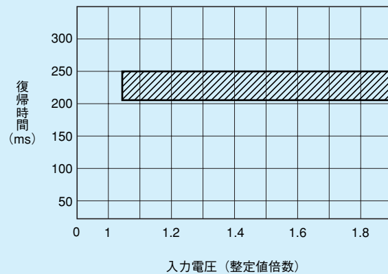
第8-4-2図 復帰時間特性
