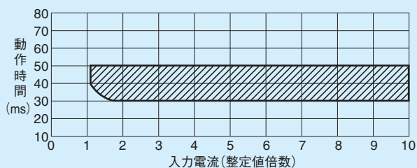
第8-2-2図 動作時間特性(瞬時要素)
