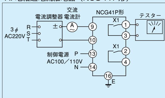
第12-6-1図 動作値試験回路
