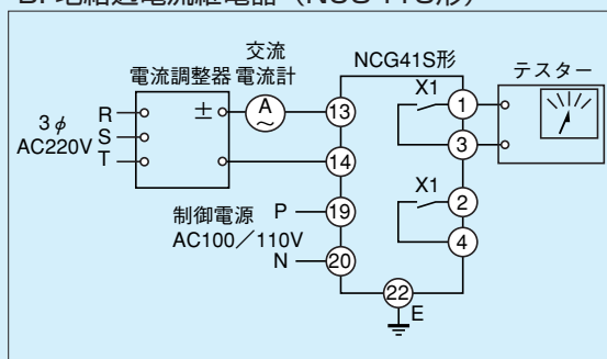
第12-6-3図 動作値試験回路
