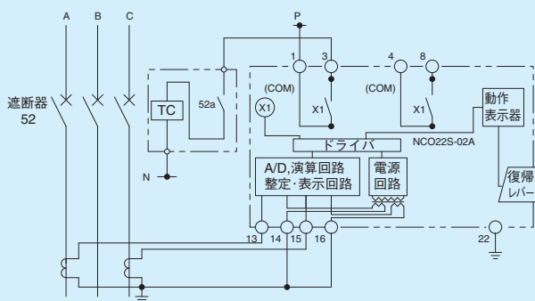
第8-1-3図 NC022S形 外部接続図
