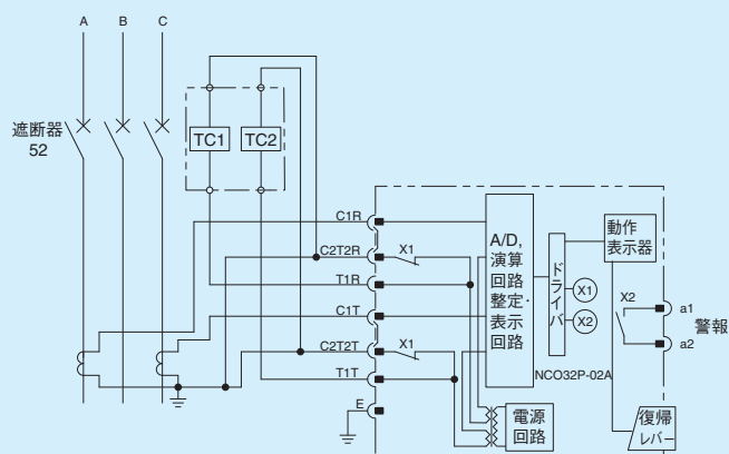
第8-2-4図 NC032P形 外部接続図
