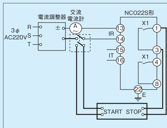
第12-2-2図 時間特性試験回路
