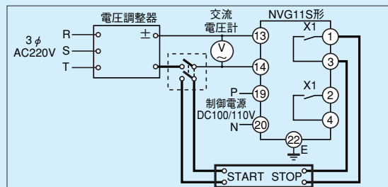
第11-7-4図 時間特性試験回路
