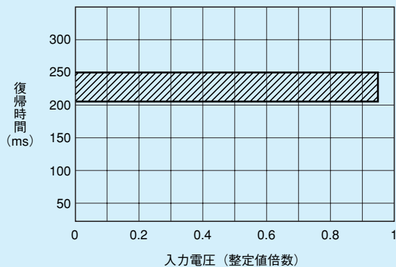
第7-5-2図 復帰時間特性
