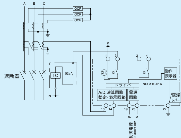
第7-6-6図 三次巻線付CT方式による地絡保護接続図例 (接続図はNCG11Sを例として使用)
