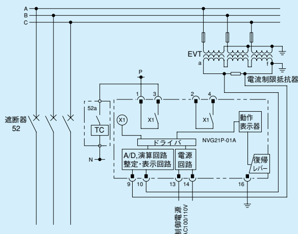
第8-6-4図 NVG21P形 外部接続図
