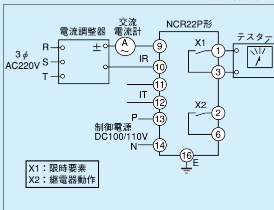
第11-3-5図 動作値試験回路
