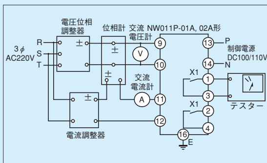
第11-10-1図 動作値試験回路
