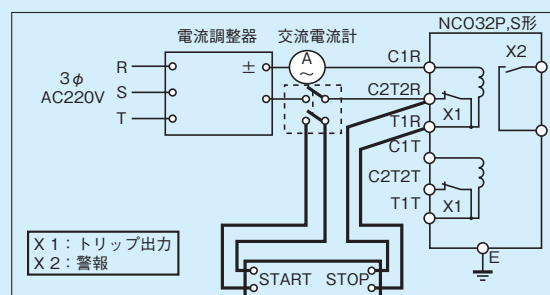
第12-3-2図 時間特性試験回路
