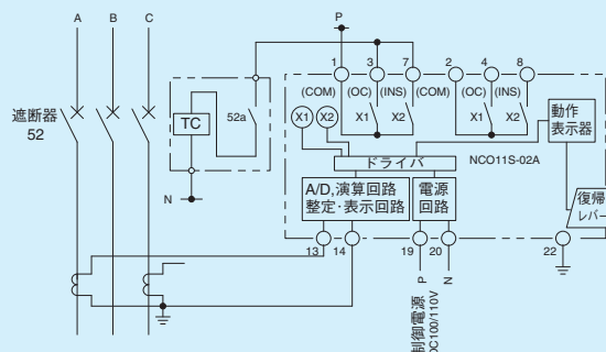
第7-1-3図 NCO11S形 外部接続図
