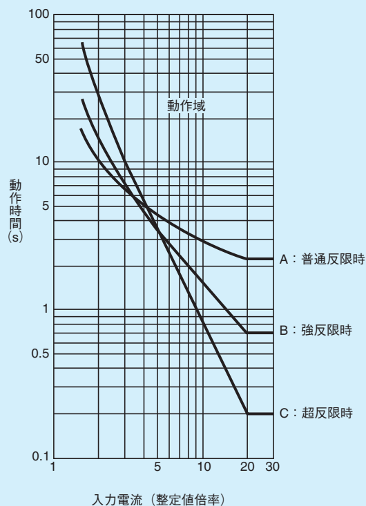
第8-1-1図 動作時間特性
