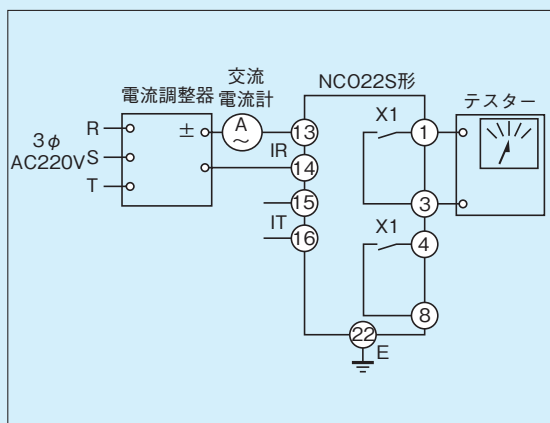
第12-2-1図 動作値試験回路
