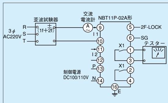
第11-9-4図 2F-LOCK試験回路
