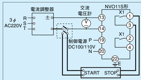
第11-4-4図 時間特性試験回路
