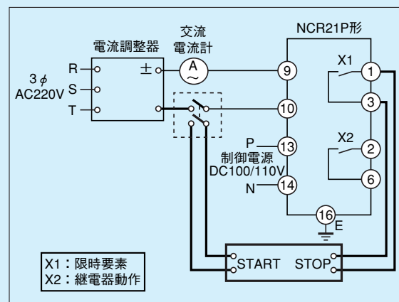
第11-3-4図 時間特性試験回路
