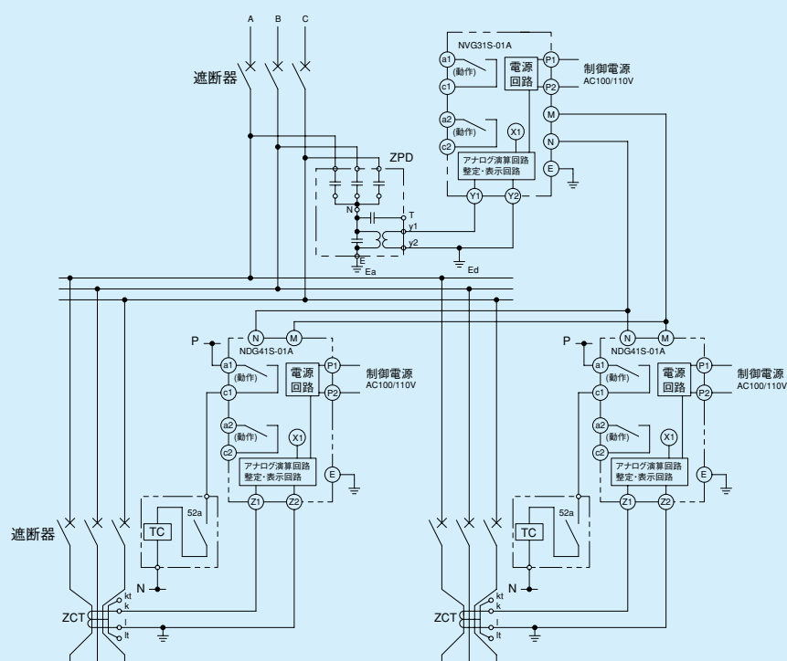
第8-7-2図 NVG31S-01A形、NDG41S-01A形 外部接続図
