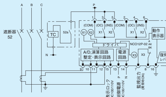
第7-1-3図 NCO11S形 外部接続図
