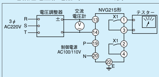
第12-7-1図 動作値試験回路
