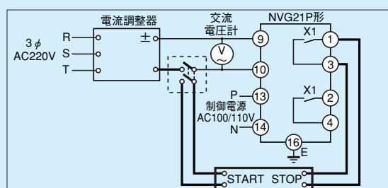
第12-7-4図 時間特性試験回路
