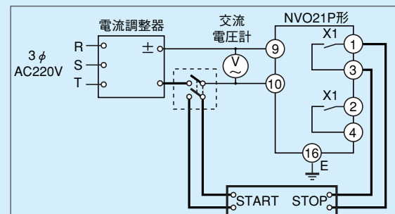
第12-4-4図 時間特性試験回路
