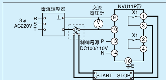
第11-5-2図 時間特性試験回路
