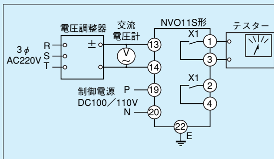
第11-4-3図 動作値試験回路
