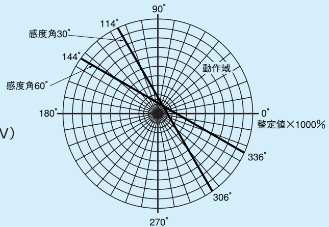
第7-7-1図 位相特性
