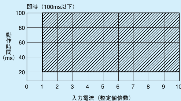
第7-7-2図 動作時間特性
