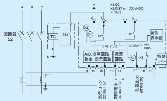
第7-2-4図 NCR21P形 外部接続図
