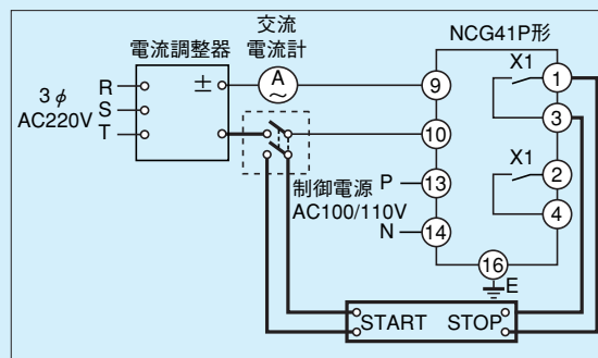
第12-6-2図 時間特性試験回路
