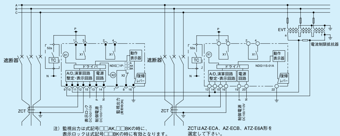
第7-7-4図 NDG11P,NDG21P,NDG11S形 外部接続図
