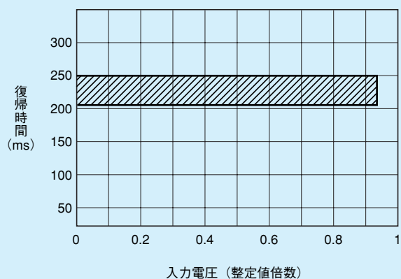
第8-3-2図 復帰時間特性
