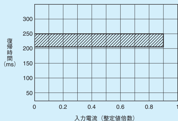
第8-5-2図 復帰時間特性
