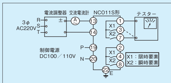
第11-2-5図 動作値試験回路
