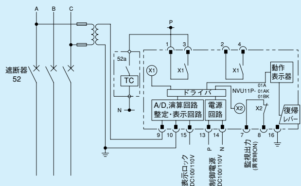
第7-4-3図 NVU11P形 外部接続図
