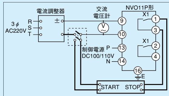
第11-4-2図 時間特性試験回路
