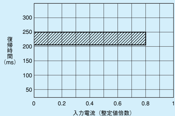
第7-7-3図 復帰時間特性
