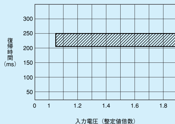
第7-4-2図 復帰時間特性
