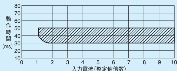
第8-1-2図 動作時間特性(瞬時要素)
