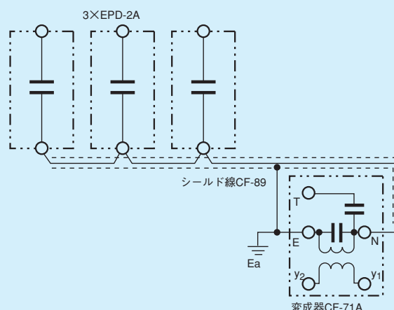
第13-2-1図 ZPC-9BS 内部接続図
