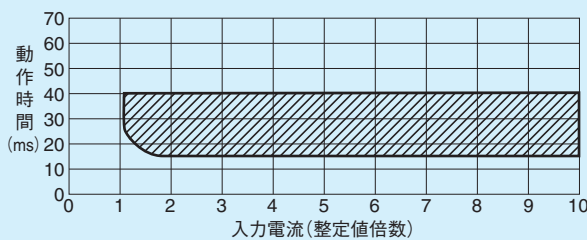
第7-2-2図 動作時間特性(瞬時要素)
