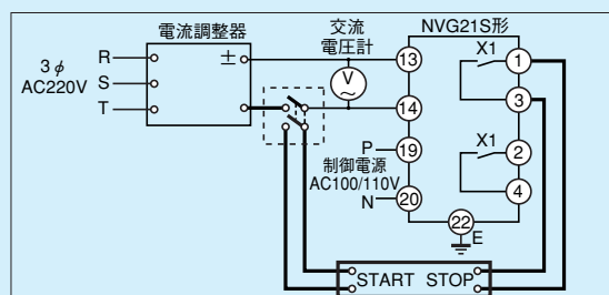
第12-7-2図 時間特性試験回路
