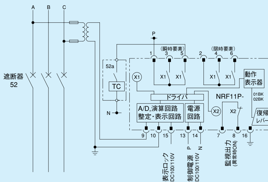
第7-10-1図 NRF11P形 外部接続図
