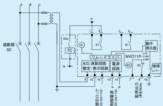
第7-3-3図 NVO11P形 外部接続図
