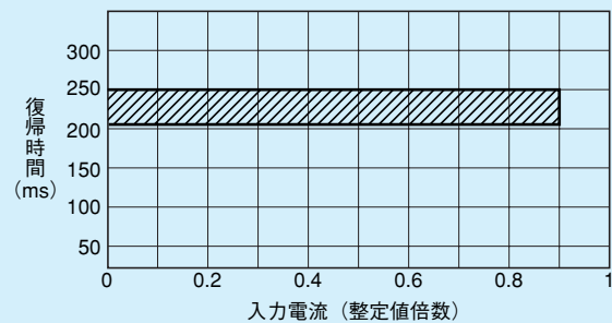
第8-8-2図 復帰時間特性
