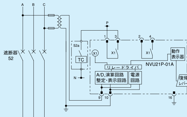
第8-4-4図 NVU21P形 外部接続図
