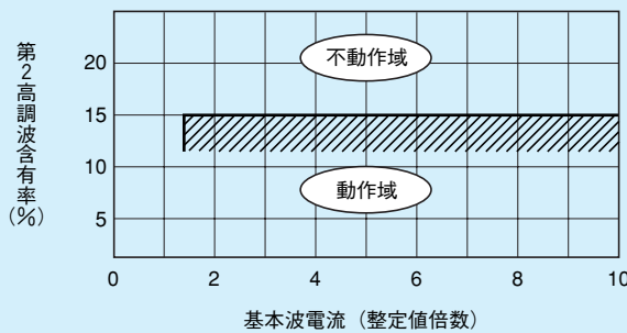
第7-6-3図 2fロック特性
