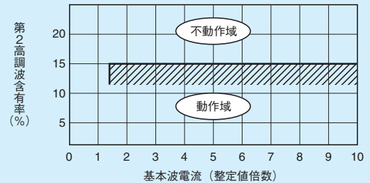
第7-9-4図 2Fロック特性
