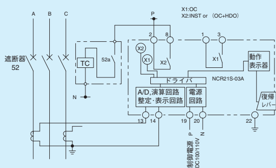
第7-2-3図 NCR21S形 外部接続図
