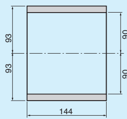
穴明図
