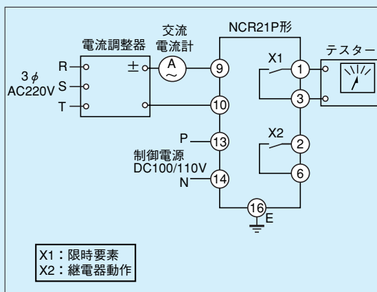
第11-3-3図 動作値試験回路
