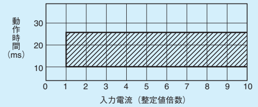
第7-9-2図 動作時間特性(HOC要素)
