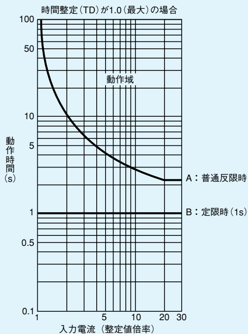
第7-8-2図 動作時間特性 (タイムダイヤル1)
