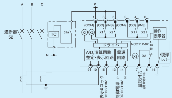
第7-1-4図 NCO11P形 外部接続図
