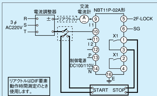
第11-9-2図 時間特性試験回路
