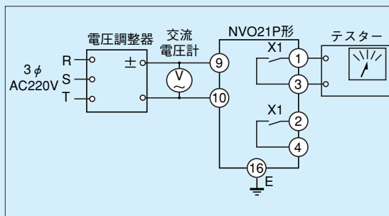
第12-4-3図 動作値試験回路
