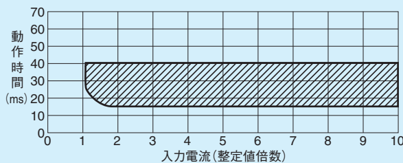
第7-1-2図 動作時間特性(瞬時要素)
