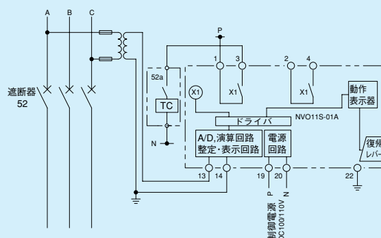
第7-3-4図 NVO11S形 外部接続図
