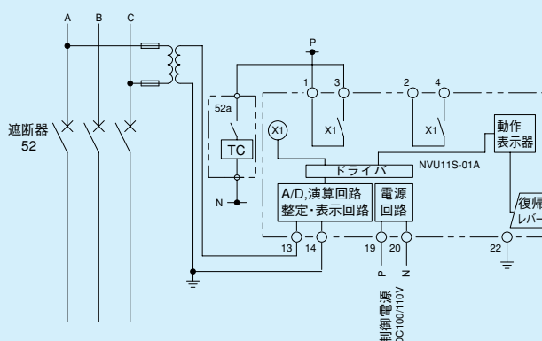
第7-4-4図 NVU11S形 外部接続図
