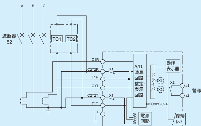
第8-2-3図 NC032S 外部接続図
