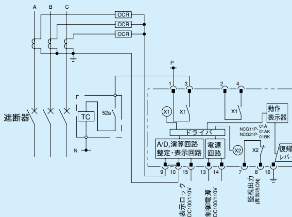
第7-6-5図 残留回路方式による地絡保護接続図例 (接続図はNCG11P,21Pを例として使用)
