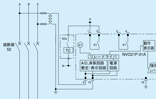
第8-3-4図 NVO21P形 外部接続図
