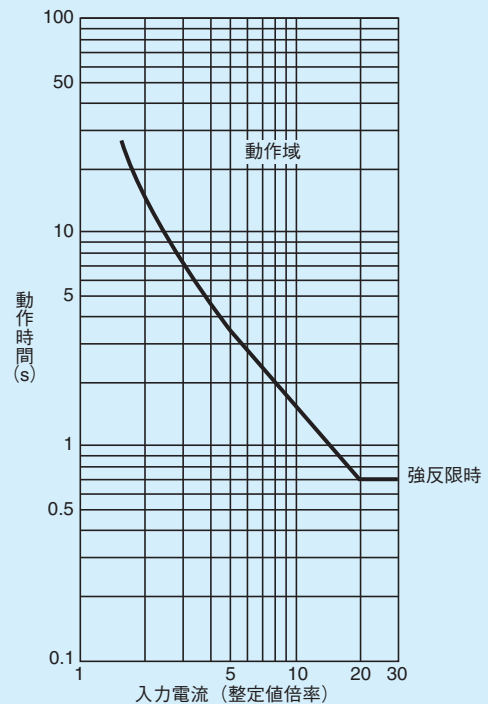
第7-2-1図 動作時間特性(限時要素) (タイムダイヤル1)
