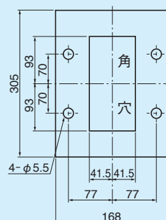
NRAD-02A(D-2ケース互換用)外形図
