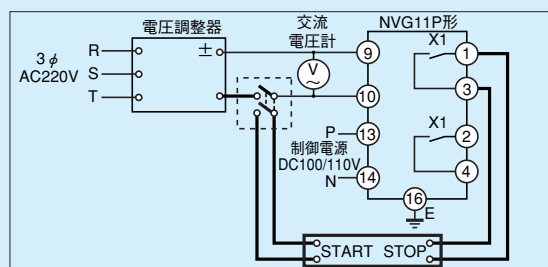
第11-7-2図 時間特性試験回路
