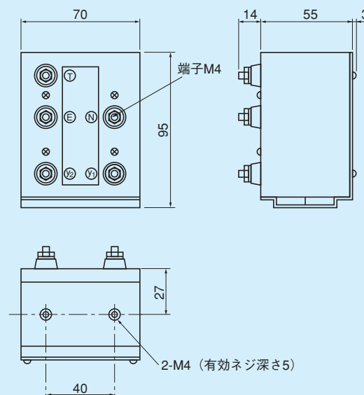
(b) 変成器CF-71A詳細図
