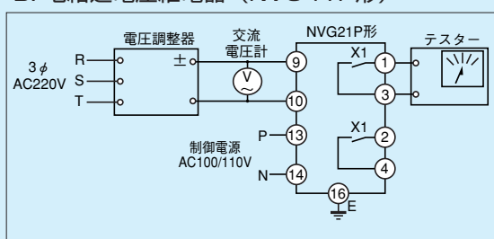
第12-7-3図 動作値試験回路
