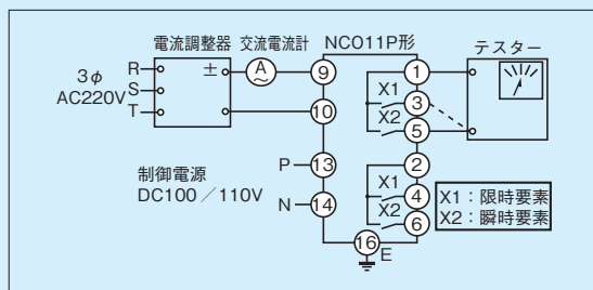
第11-2-1図 動作値試験回路
