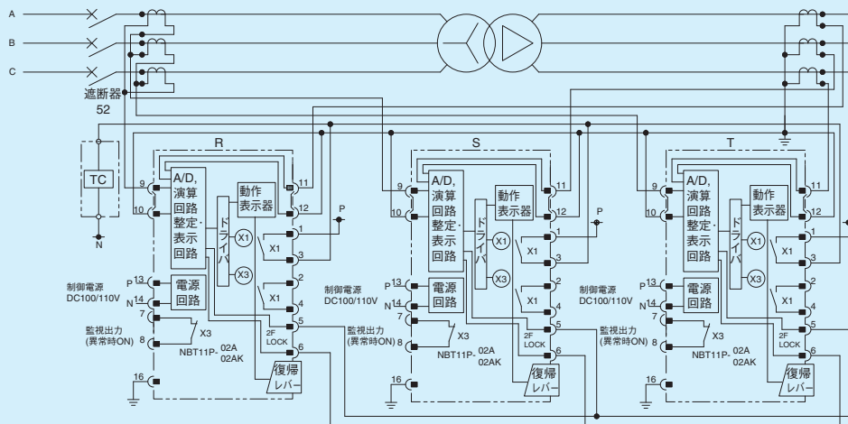
第7-9-6図 NBT11P形 外部接続図
