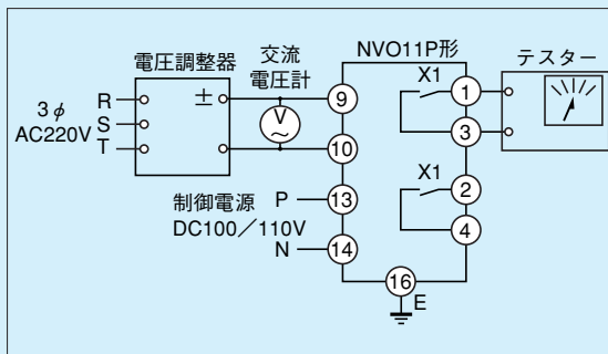
第11-4-1図 動作値試験回路
