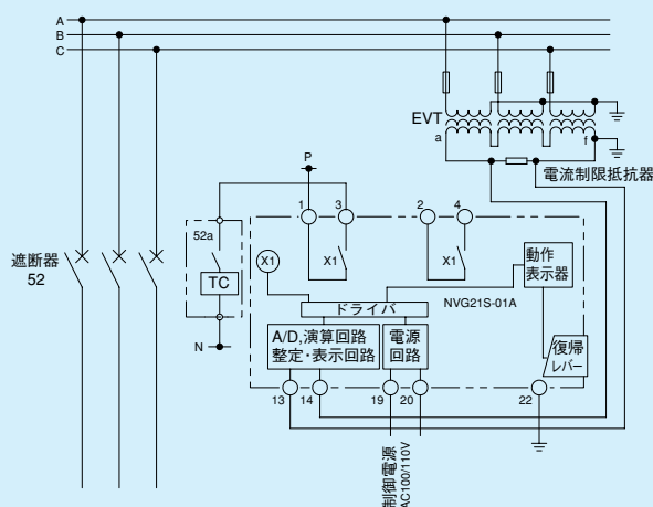
第8-6-3図 NVG21S形 外部接続図
