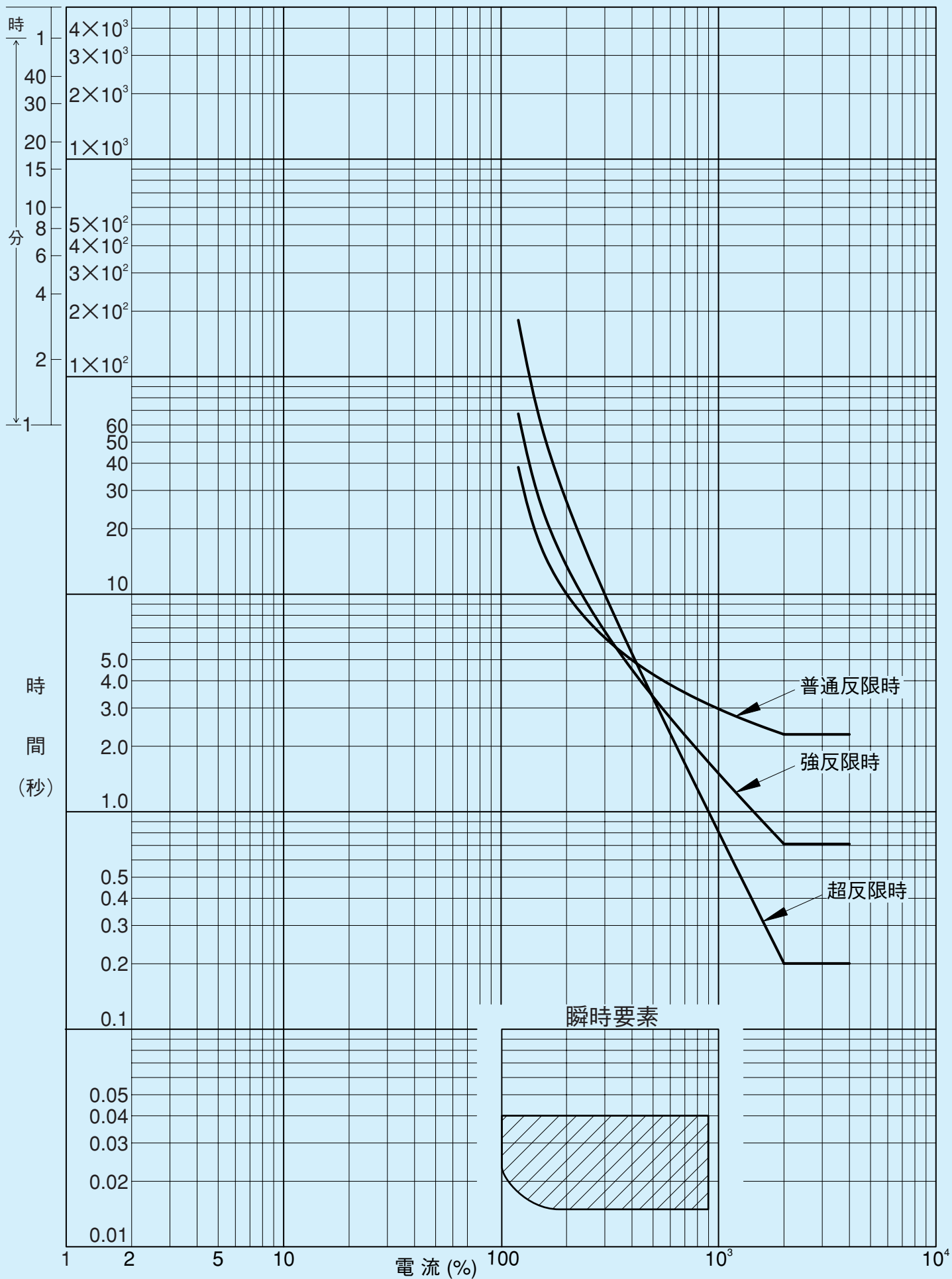
第14-1-1図 NCO1□□形 動作時間特性例
