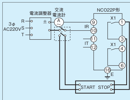
第12-2-4図 時間特性試験回路
