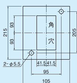
外形図
