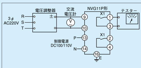
第11-7-1図 動作値試験回路
