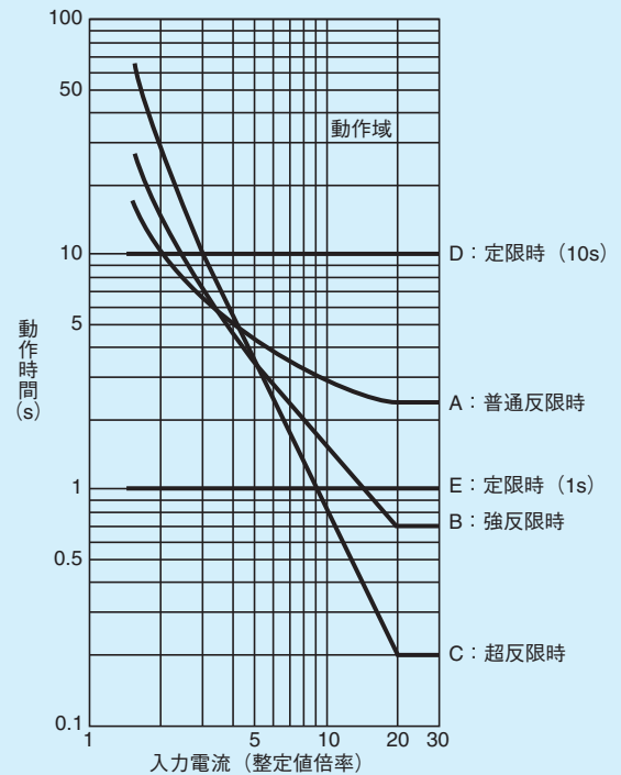
第7-1-1図 動作時間特性(限時要素) (タイムダイヤル1)
