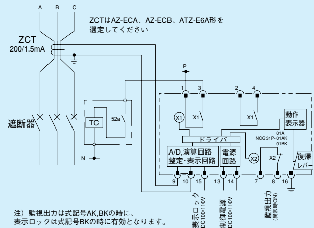
第7-6-4図 ZCT方式による地絡保護接続図例 (NCG31P)
