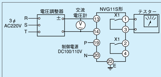
第11-7-3図 動作値試験回路
