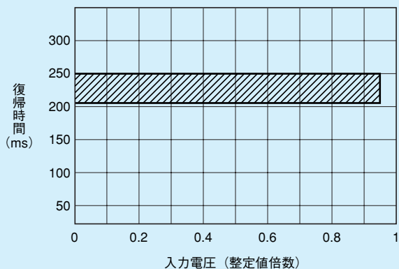
第8-6-2図 復歸時間特性
