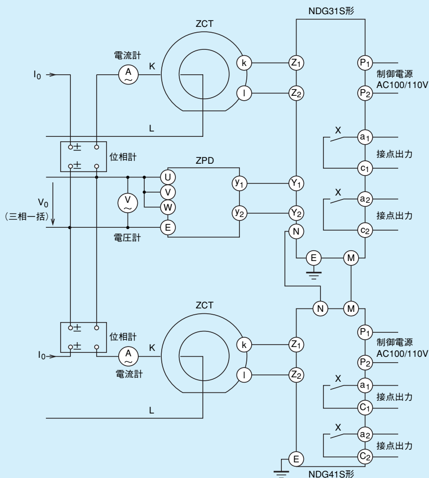
第12-9-1図 試験回路
