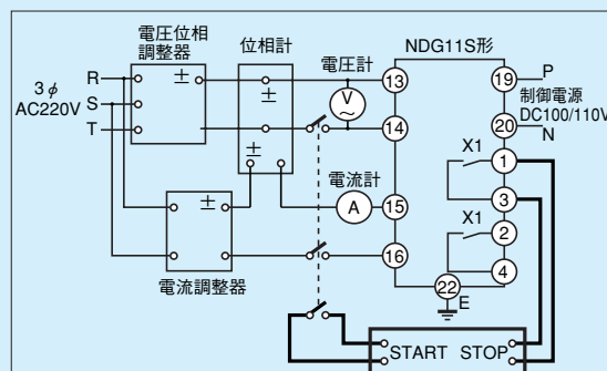
第11-8-4図 時間特性試験回路
