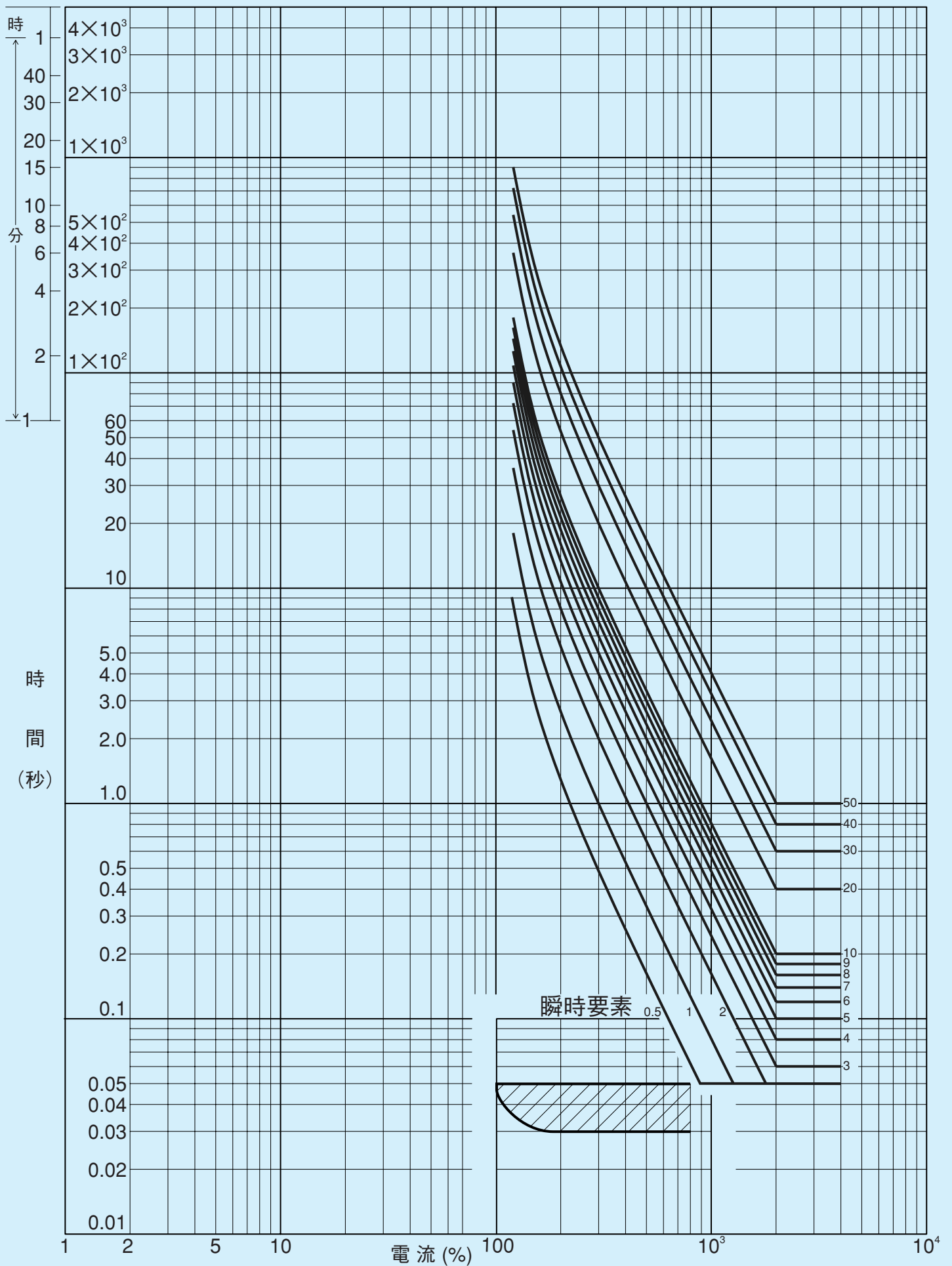
第14-1-3図 NCO32□形 動作時間特性例
