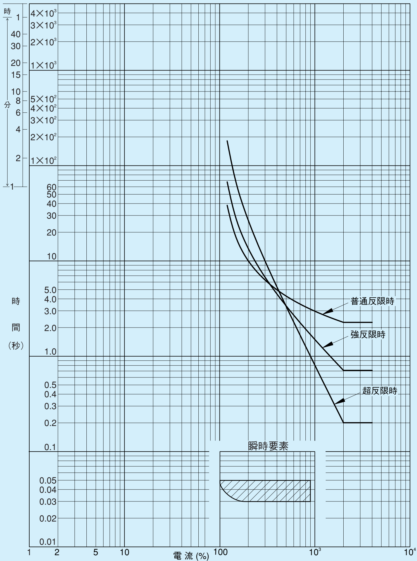
第14-1-2図 NCO22□形 動作時間特性例
