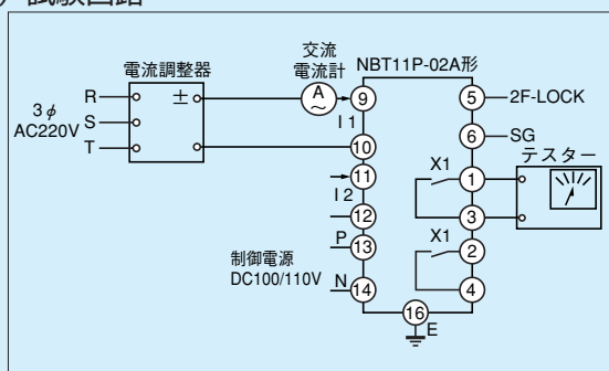
第11-9-1図 動作値試験回路
