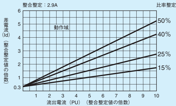
第7-9-3図 比率特性
