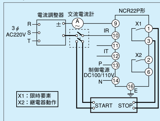
第11-3-6図 時間特性試験回路
