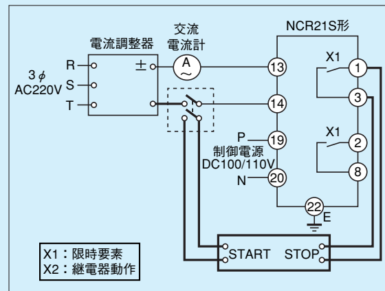
第11-3-2図 時間特性試験回路
