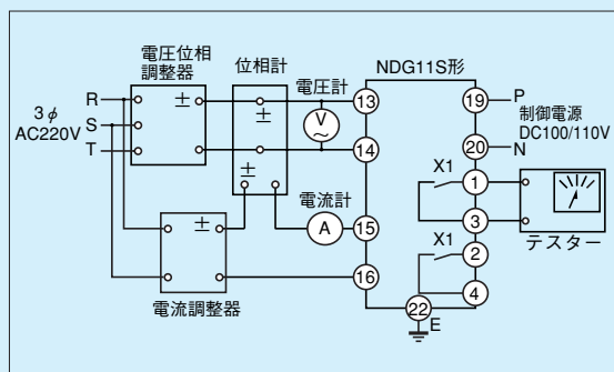
第11-8-3図 動作値試験回路
