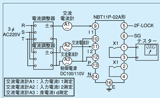
第11-9-3図 比率特性試験回路
