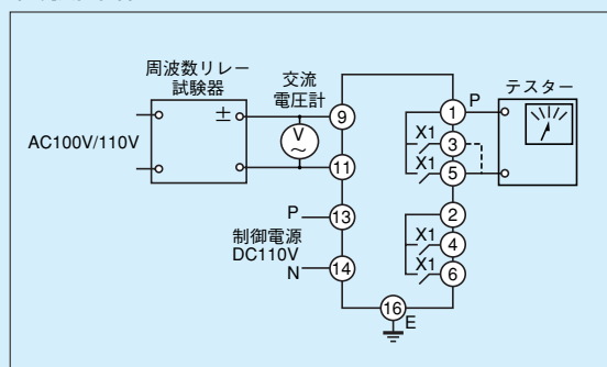
第11-11-1図 動作値試験回路
