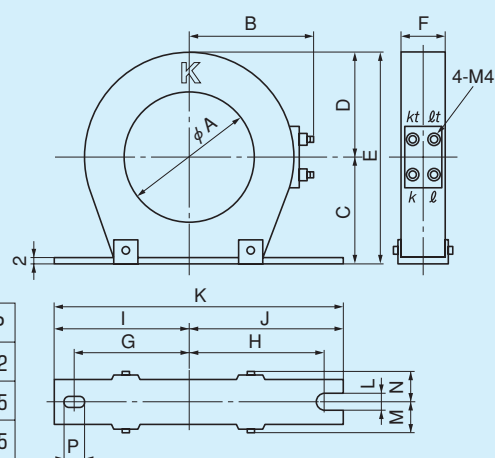
第13-3-1図 零相変流器外形および接続図
