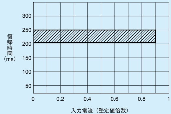
第7-6-2図 復帰時間特性
