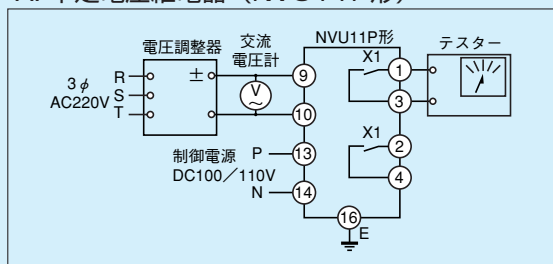
第11-5-1図 動作値試験回路
