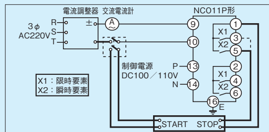
第11-2-2図 時間特性試験回路
