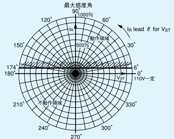
第7-8-1図 位相特性
