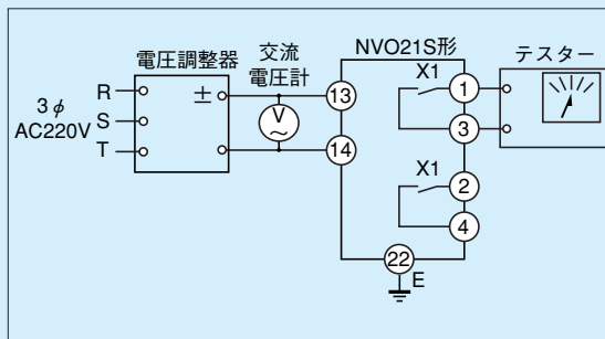
第12-4-1 動作値試験回路
