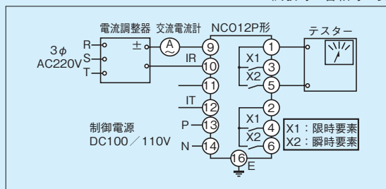
第11-2-3図 動作値試験回路
