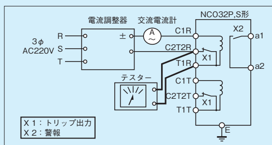
第12-3-1図 動作値試験回路
