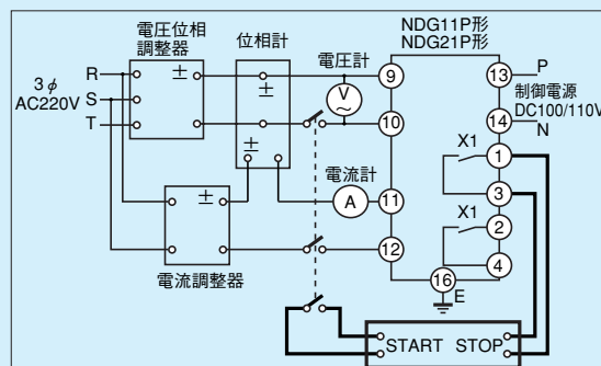
第11-8-2図 時間特性試験回路
