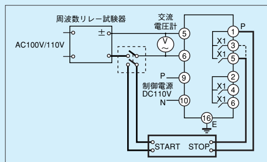
第11-11-2図 時間特性試験回路
