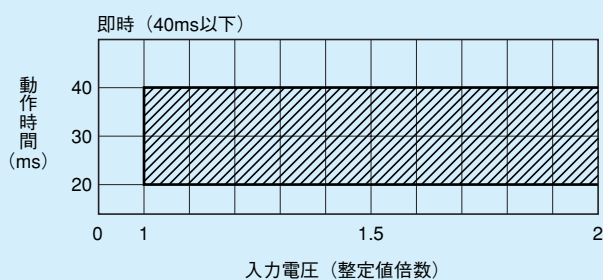
第8-6-1図 動作時間特性
