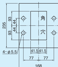
NRAD-01A(D-1ケース互換用)外形図
