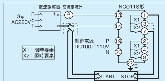
第11-2-6図 時間特性試験回路
