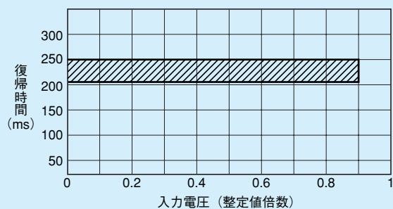
第8-7-1図 復帰時間特性
