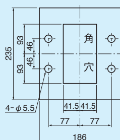
外形図
