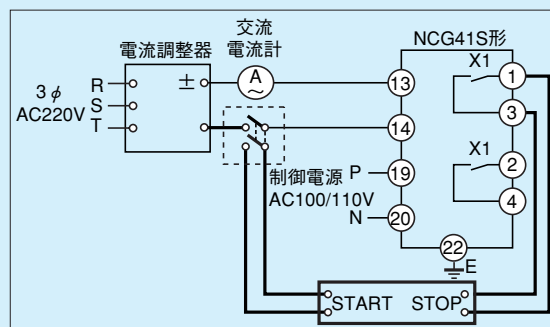
第12-6-4図 時間特性試験回路
