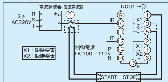
第11-2-4図 時間特性試験回路
