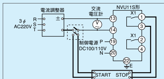
第11-5-4図 時間特性試験回路
