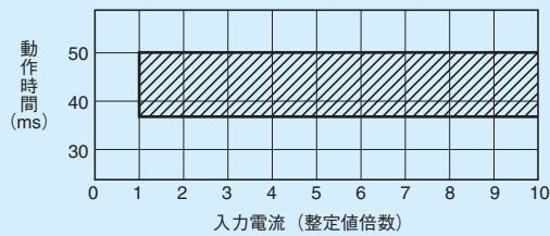
第7-9-1図 動作時間特性(DIF要素)
