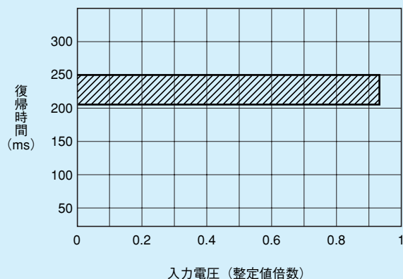
第7-3-2図 復帰時間特性
