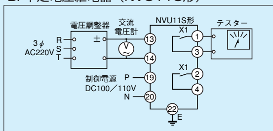
第11-5-3図 動作値試験回路
