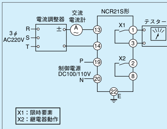
第11-3-1図 動作値試験回路
