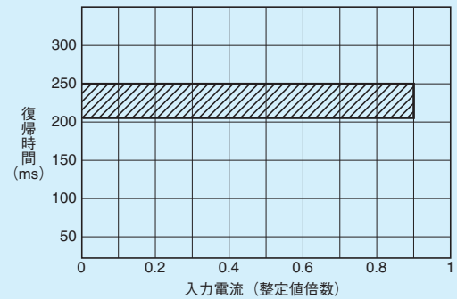
第7-9-5図 復帰時間特性
